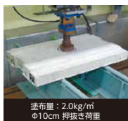
塗布量: 2.0kg/m 2 φ10cm 押抜き荷重
