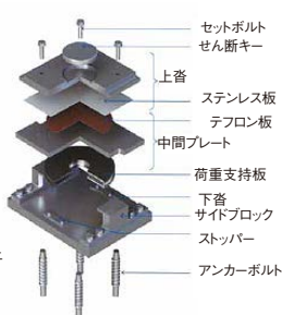
可動支承
